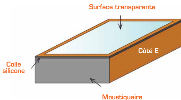
↑ Capteur solaire
